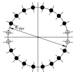
DN 450-600
