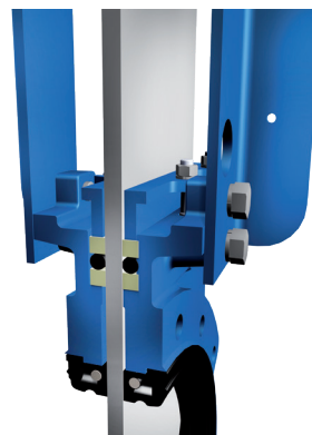
(Fig. 4) Option : garniture étanche conventionnelle
