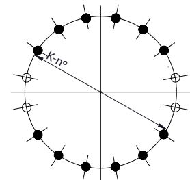
DN 350-400
